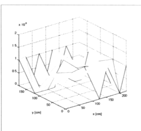
Fig. 7 - Interpolazione planare dei tempi di ritorno degli impulsi significativi al di fuori del recinto del teatro (quadrato C)
