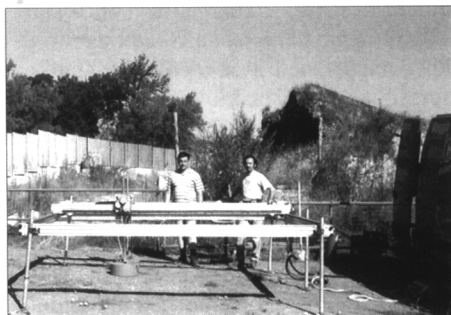
Fig. 2 - Immagine dello strumento: in primo piano c'è il sistema di posizionamento con sopra le antenne, il rack è a bordo del furgone sulla destra.
