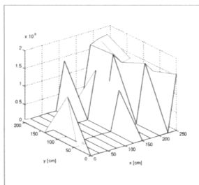
Fig. 4 - Interpolazione planare dei tempi di ritorno degli impulsi significativi sulla strada romana (quadrato A).
